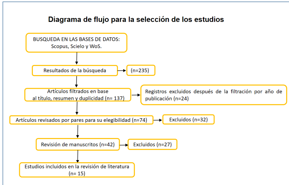
Figura 1. Declaración PRISMA.
